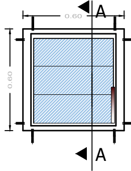
ELEVACION
