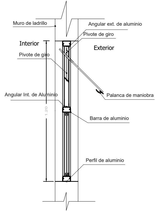
SECCION A-A
