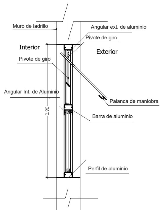
SECCION A-A
