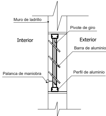
SECCION A-A
