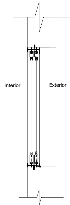
SECCION A-A
