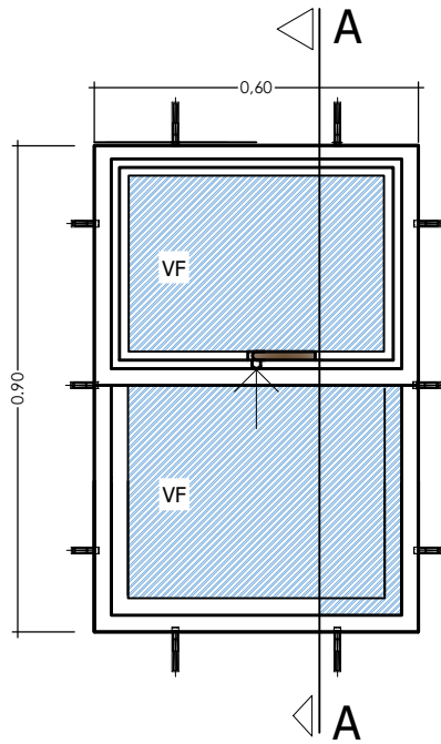
ELEVACION
