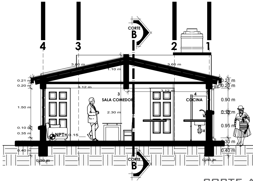
CORTE A-A
