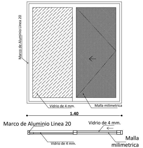
Ventana Tipo 2
