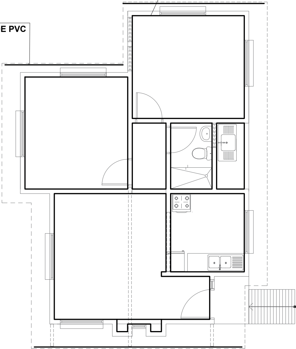
PLANO DE PVC INTERIOR - EXTERIOR ESC. 1:75
