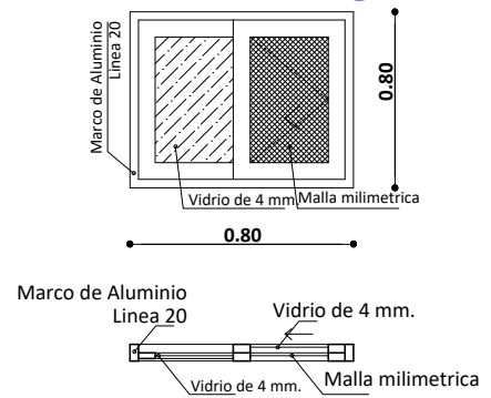
Ventana Tipo 3
