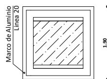
Ventana Tipo 4
