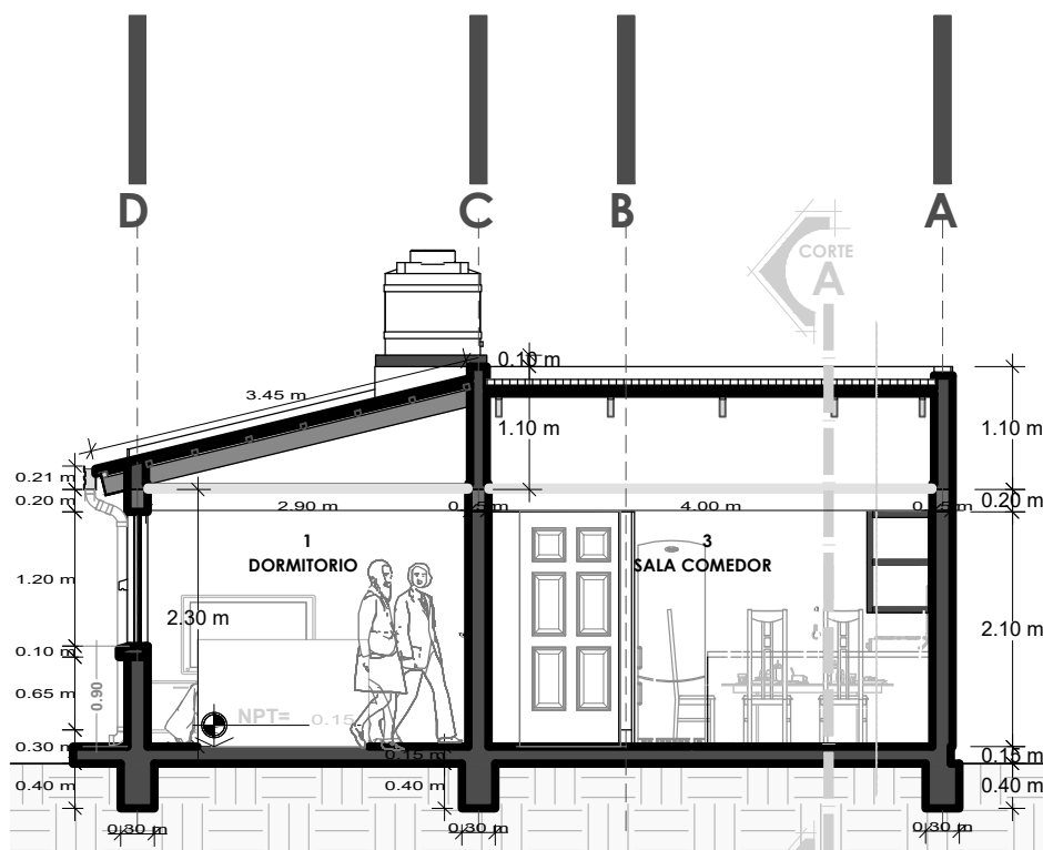
CORTE B-B'
