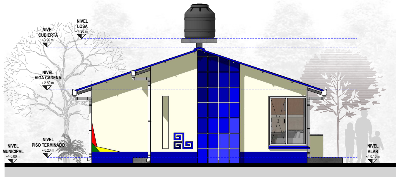
TIPO 3 FRONTAL ESC. 1:75
