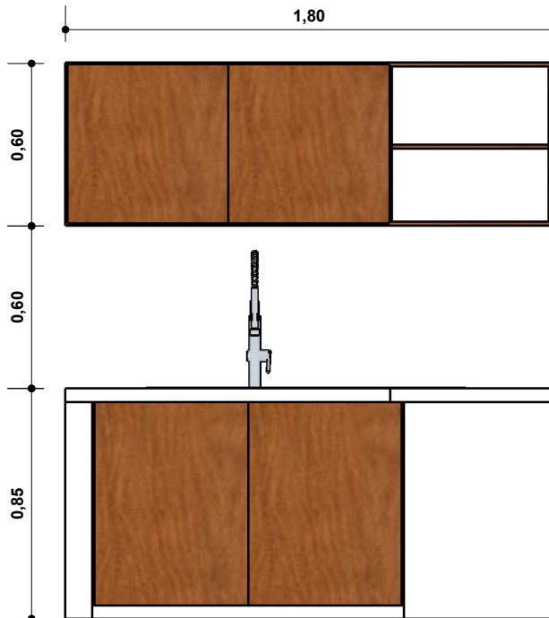
ELEVACION
