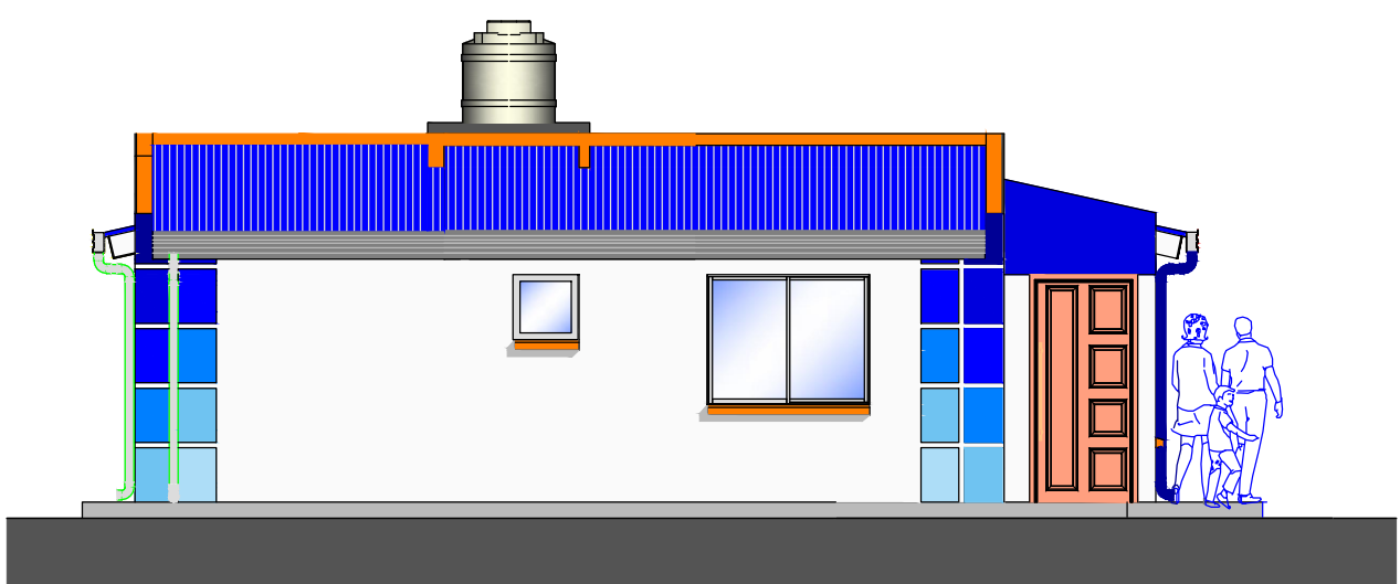
ELEVACION LATERAL
