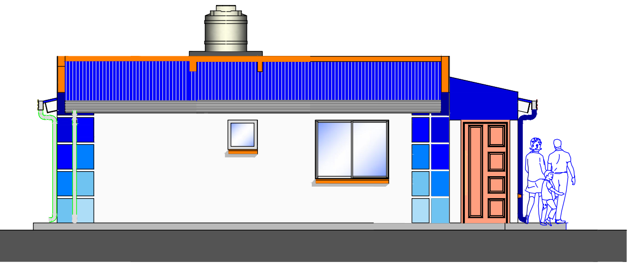
ELEVACION LATERAL
