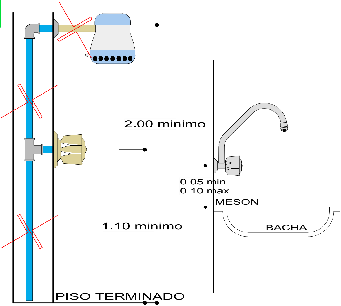
DETALLE DE DUCHA ESCALA: 1:20
