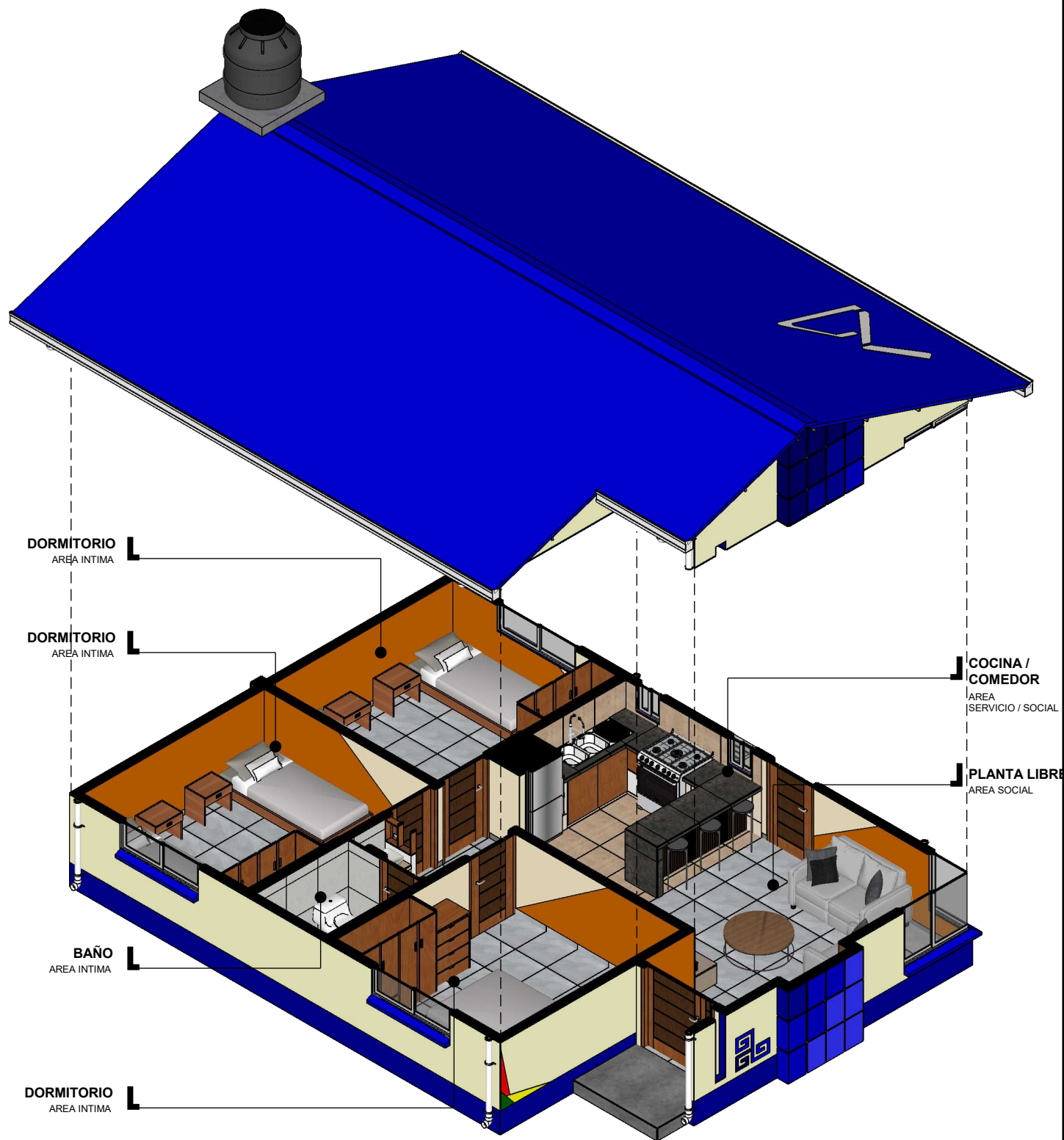
TIPO 3 PLANTA ISOMETRICA ESC. 1:75
