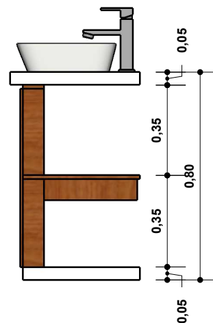
ELEVACION LATERAL
