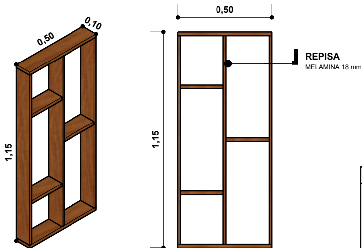
ISOMETRIA REPISA DE MELAMINA MAS ACCESORIOS
