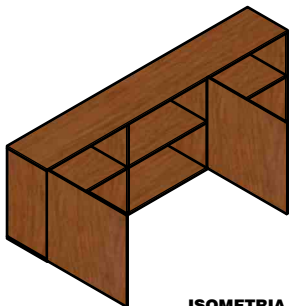
ISOMETRIA CAJONERÍA ALTA DE MELAMINA 18 mm COCINA
