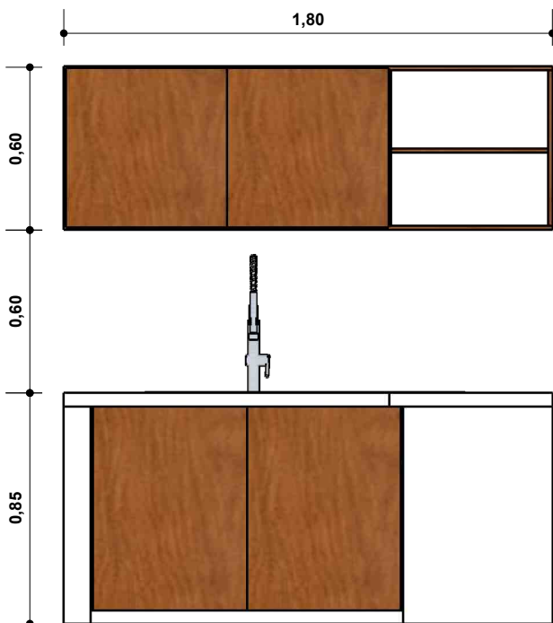
ELEVACION
