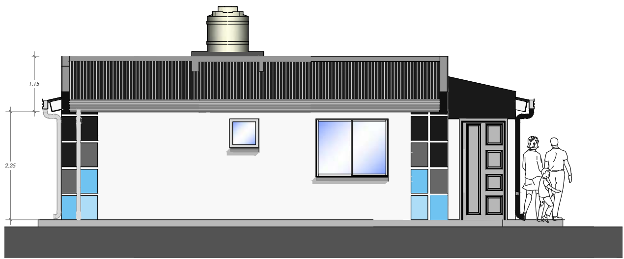
ELEVACION LATERAL
