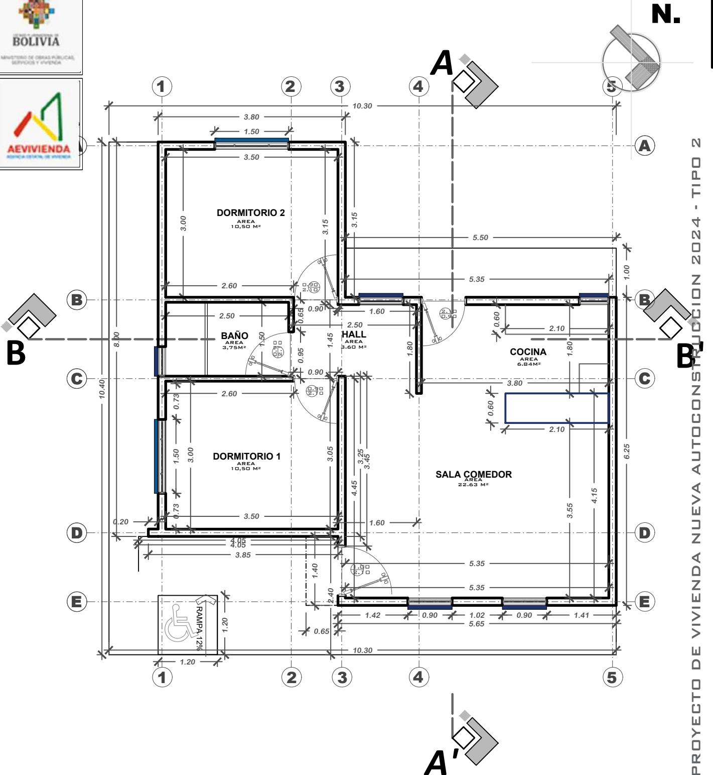
PLANTA ACOTADA
