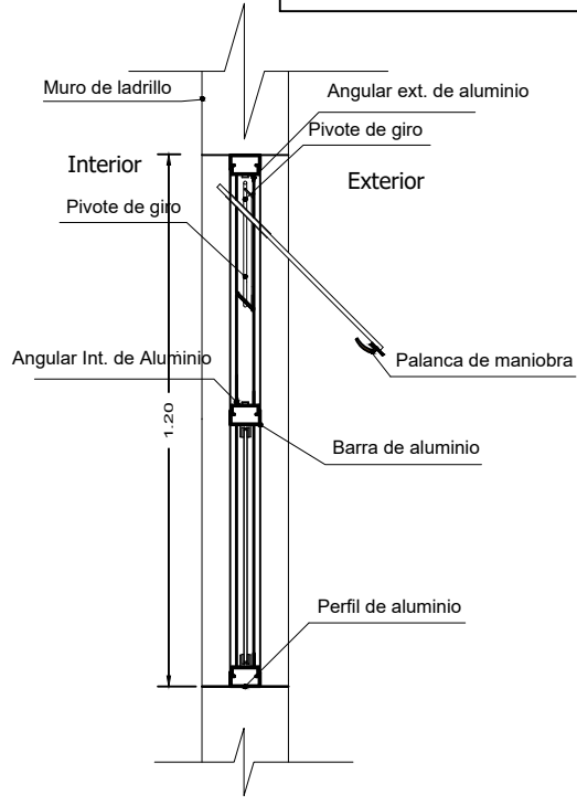
SECCION A-A
