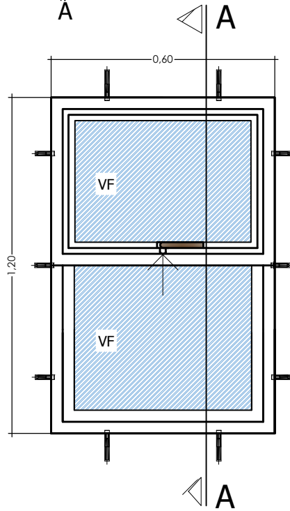
ELEVACION
