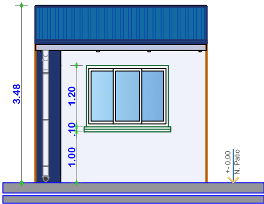
ELEVACION FRONTAL ESCALA: 1:75
