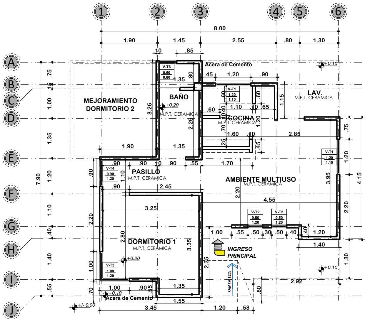
PLANTA ACOTADA ESCALA: 1:75
