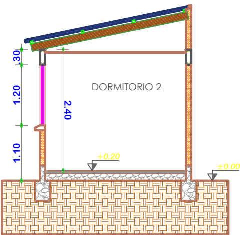
CORTE B-B' ESCALA: 1:75
