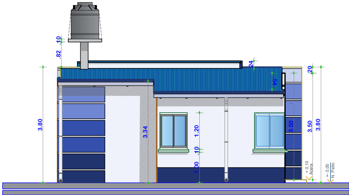
ELEVACION LATERAL IZQUIERDO ESCALA: 1:75
