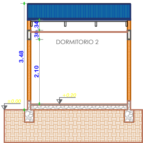
CORTE A-A' ESCALA: 1:75
