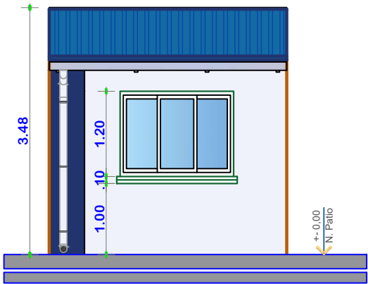
ELEVACION FRONTAL ESCALA: 1:75
