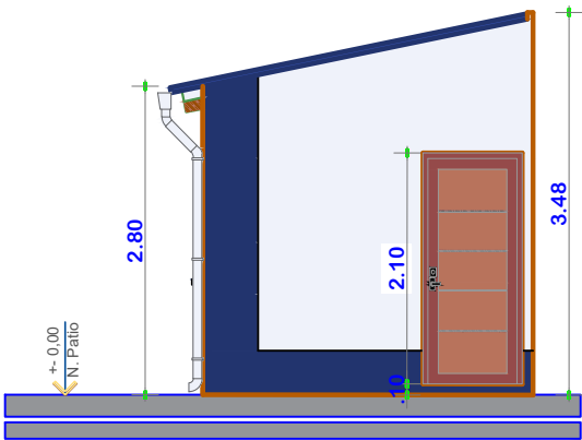
ELEVACION LATERAL ESCALA: 1:75
