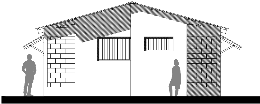
ELEVACION FRONTAL ESC. 1:75
