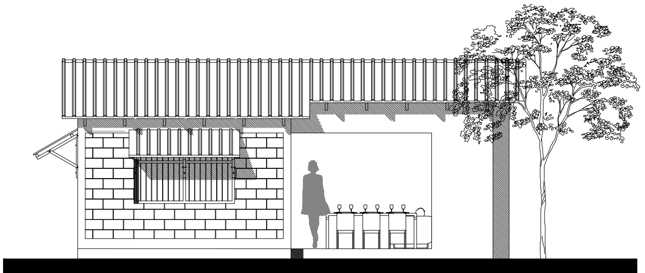
ELEVACION LATERAL ESC. 1:75
