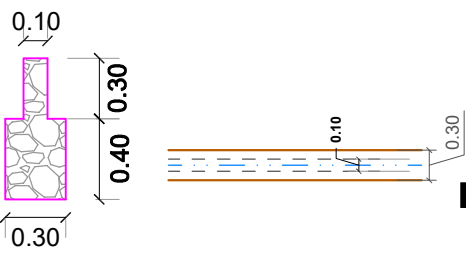
PLANTA DE SOBRECIMIENTOS ESCALA: 1:75
