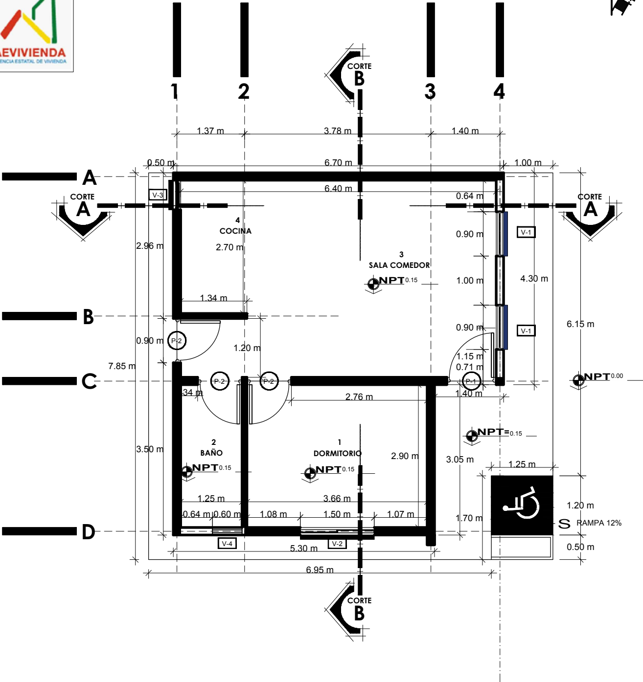
PLANO DE PLANTA ACOTADA
