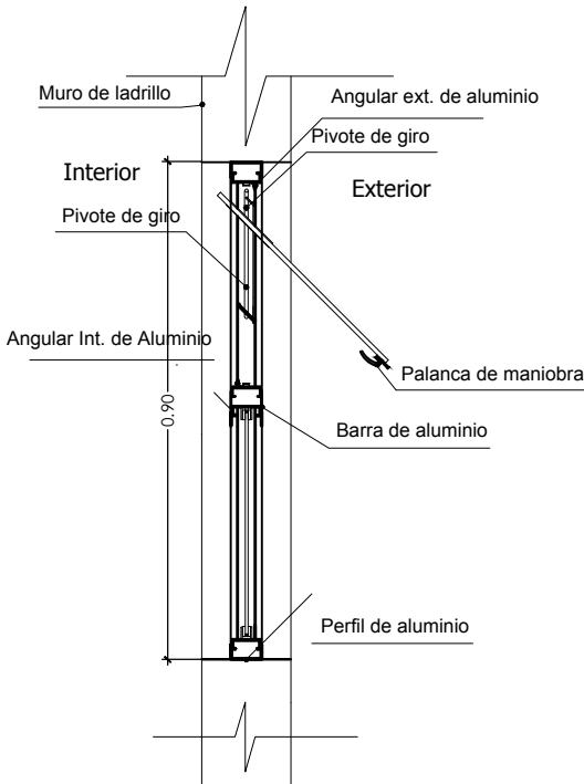
SECCION A-A
