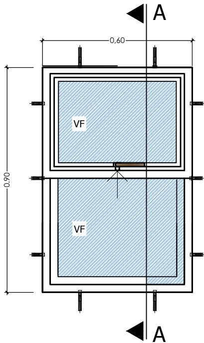
ELEVACION ELEVACION
