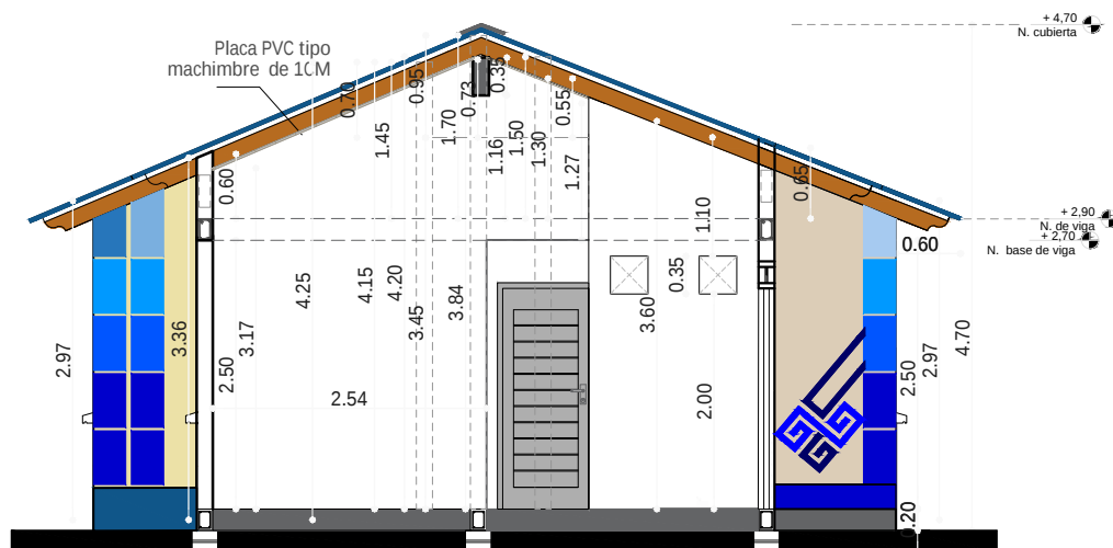
CORTE D-D"
