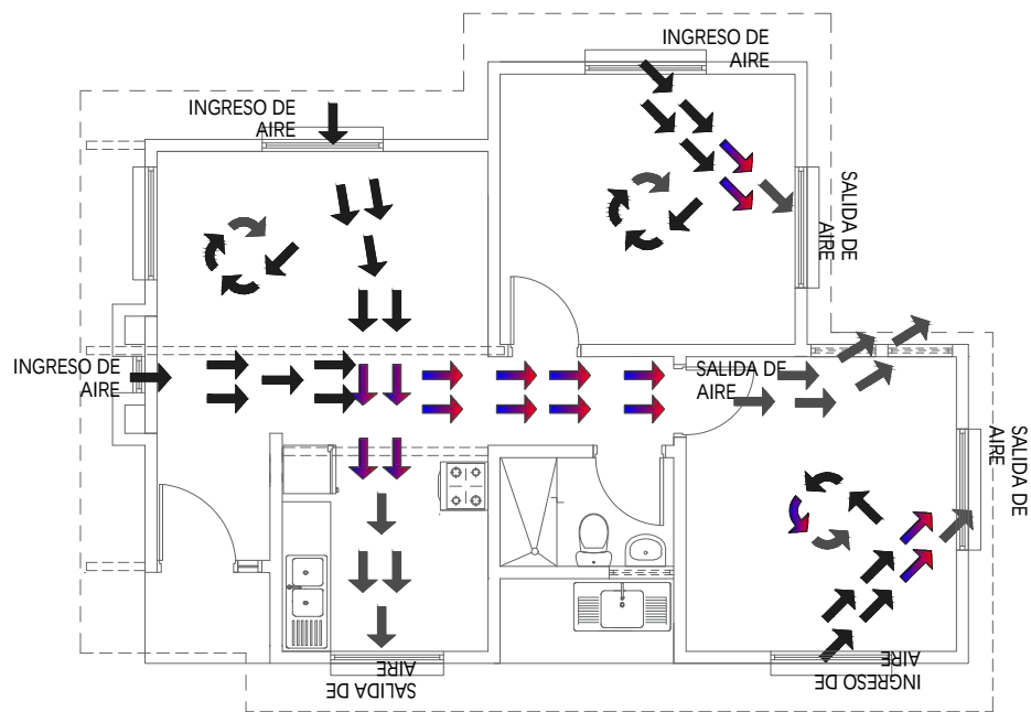
ESQUEMA PASILLO DE CIRCULACION GRUZADA ESC. 5/E
