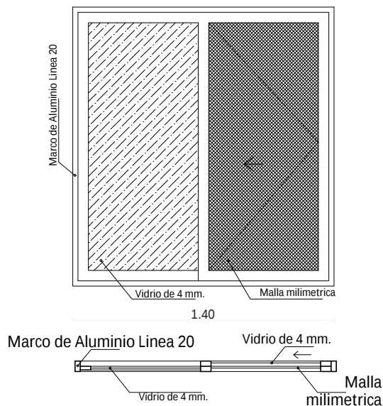
Ventana Tipo 2
