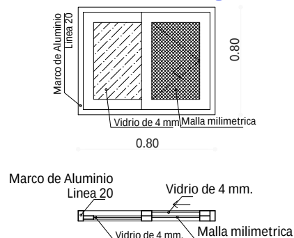
Ventana Tipo 3
