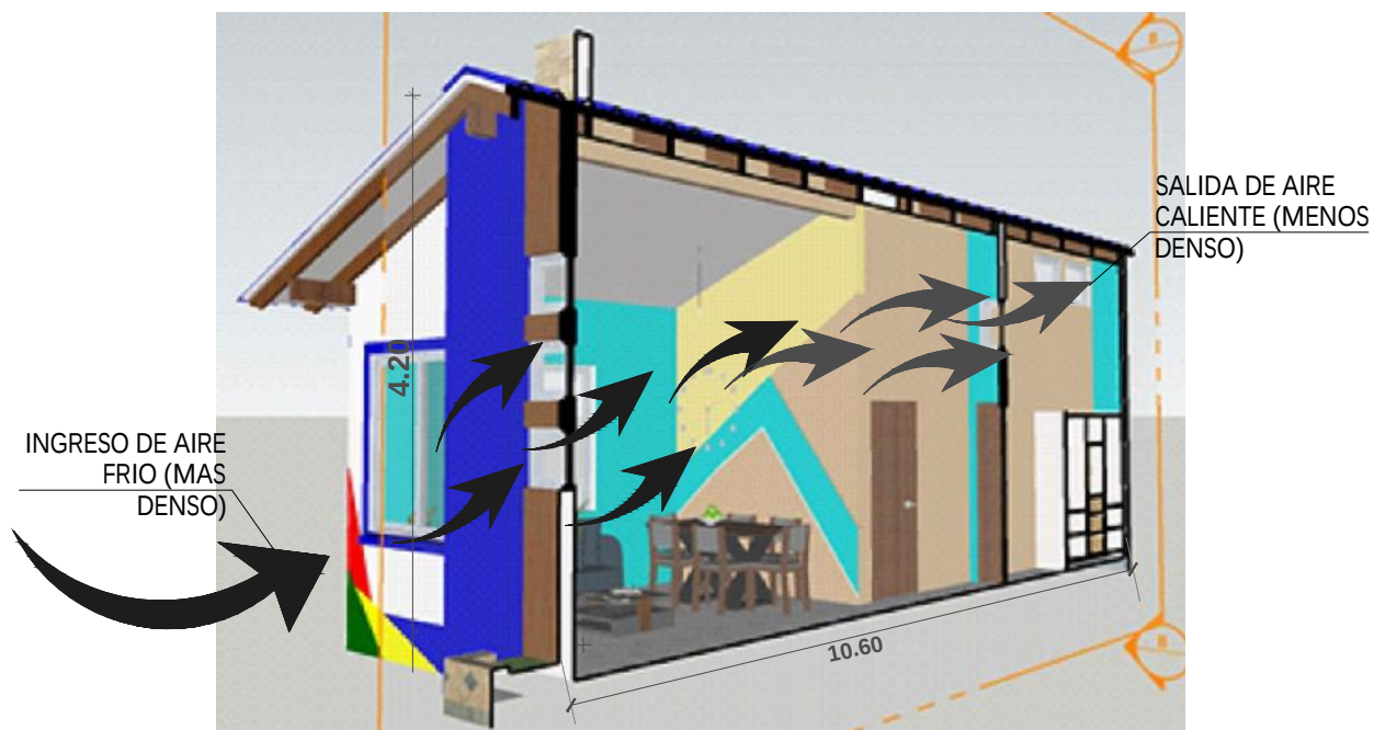
ESQUEMA PASILLO DE CIRCULACION GRUZADA ESC. 5/E
