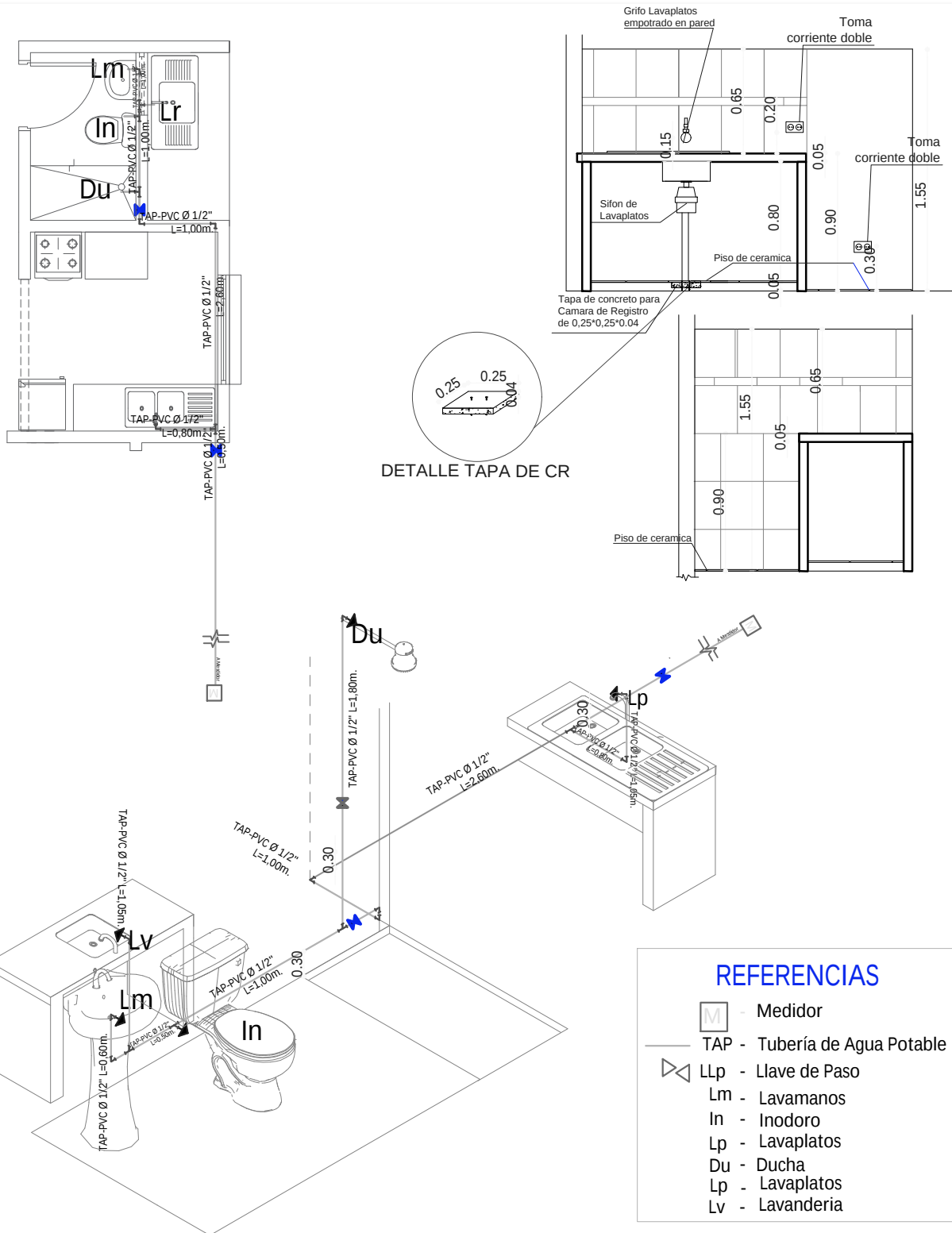
PLANO DE INSTALACION AGUA POTABLE ESC. 1:75
