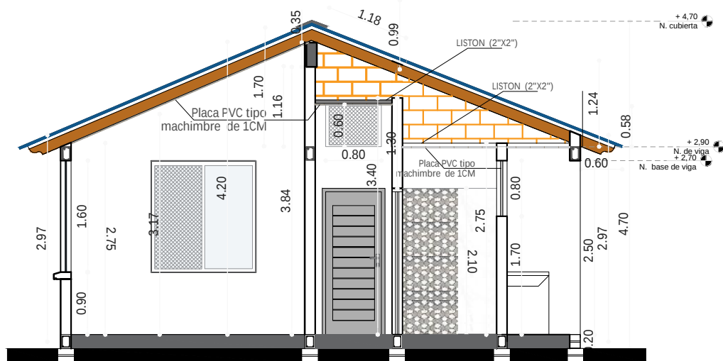
CORTE C-C"
