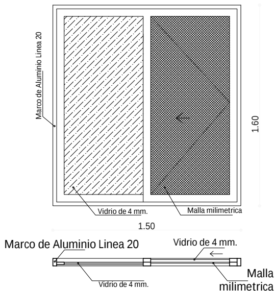
Ventana Tipo 1
