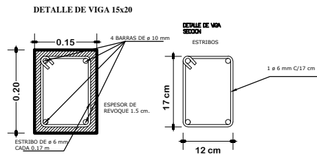
PLANTA DE VIGA DE H°A° ESCALA: 1:75
