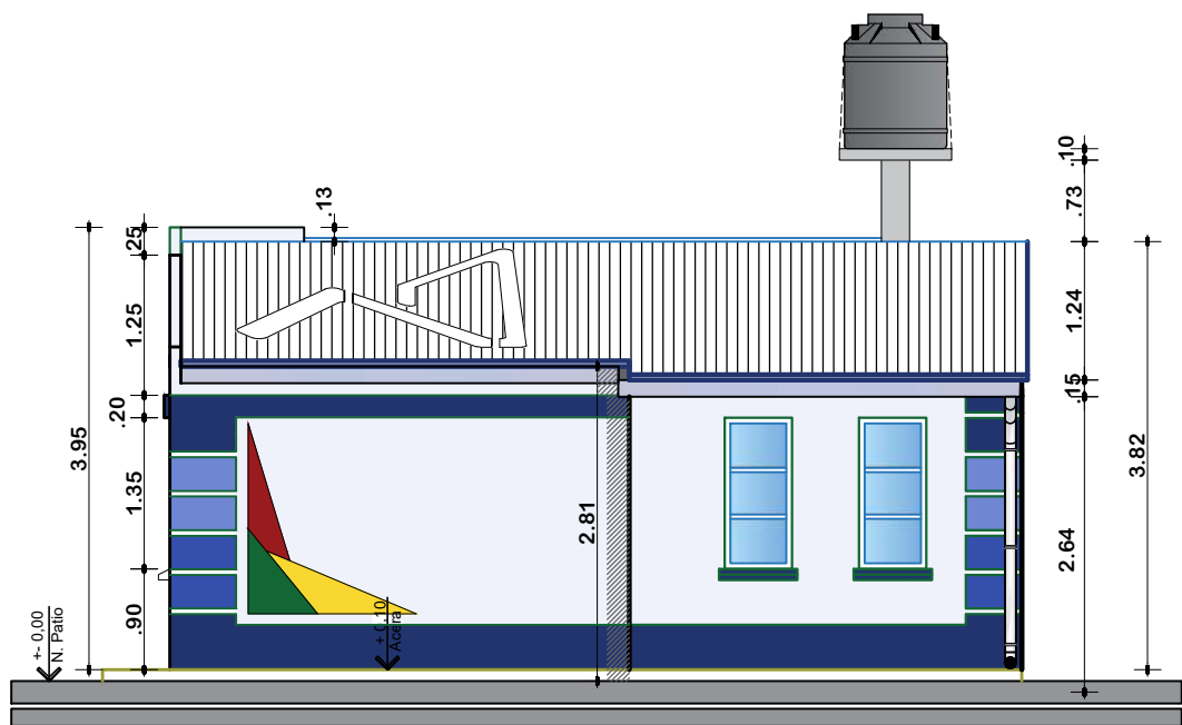
ELEVACION LATERAL IZQUIERDO ESCALA: 1:75
