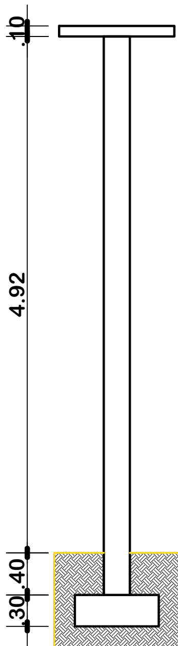
DETALLE COLUMNA DE H 0 A 0 Y ZAPATA DE H 0 A 0 ESCALA: 1:50
