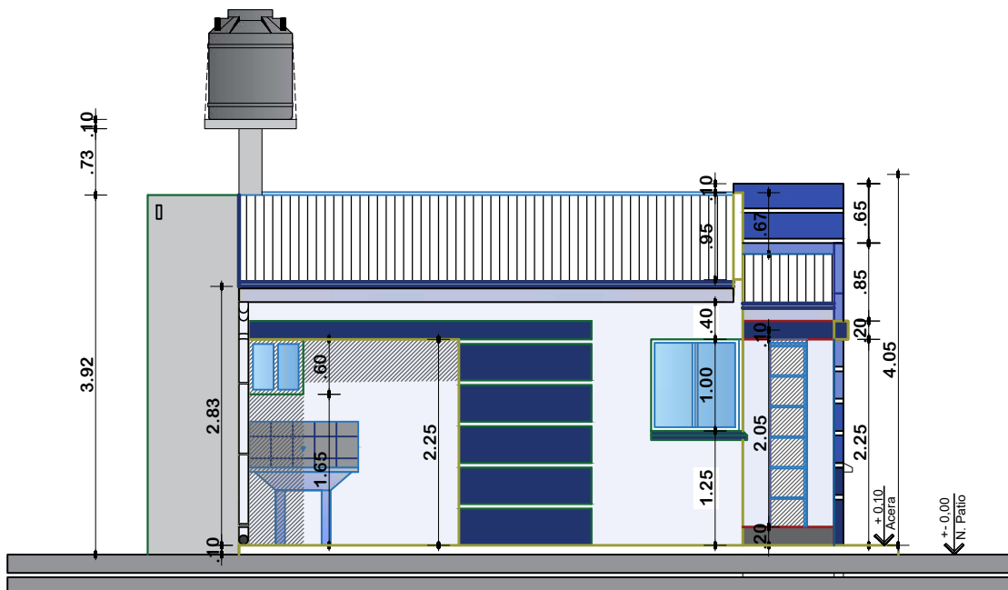
ELEVACION LATERAL DERECHO ESCALA: 1:75
