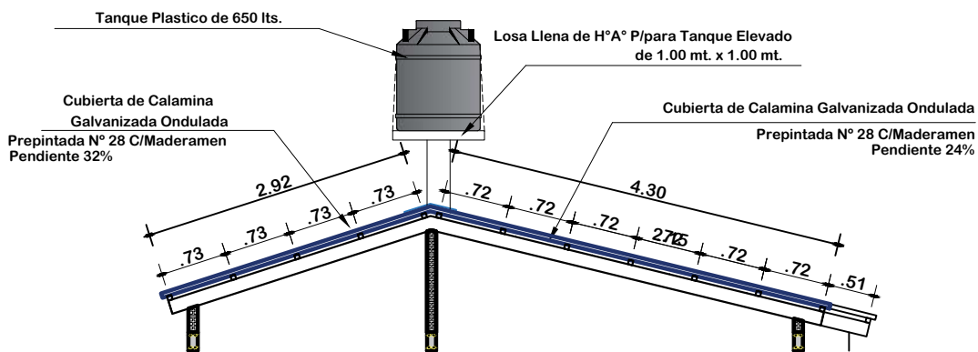
PLANO DE ESTRUCTURA MADERAMEN ESCALA: 1:75
