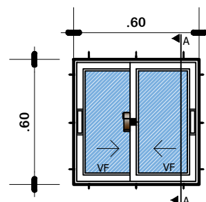
ELEVACION
