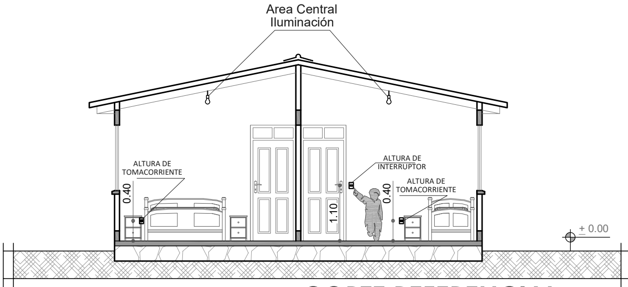
CORTE REFERENCIAL
