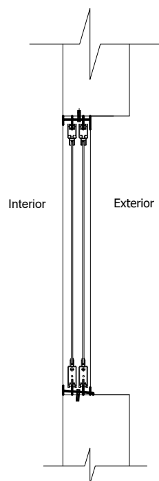
SECCION A-A
