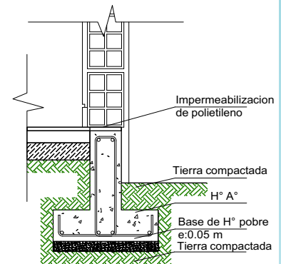
SECCIÓN ESTRIBO
