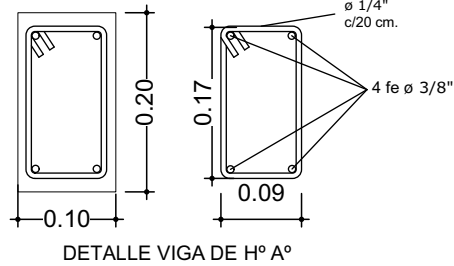
SECCION VIGA CADENA DE H°A°
