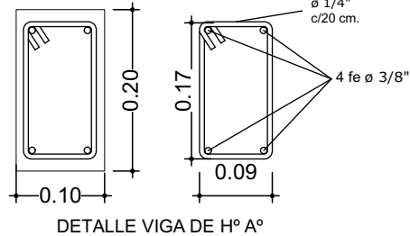
SECCION VIGA CADENA DE H°A°
