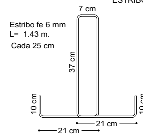
SECCION VIGA T
