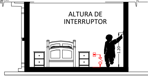
CORTE REFERENCIAL
