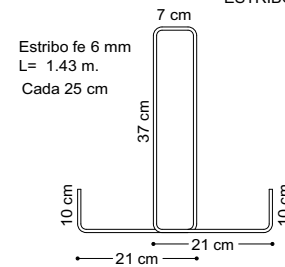
SECCIÓN VIGA T
