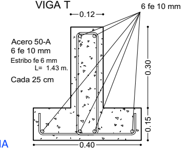
SECCIÓN VIGA T
