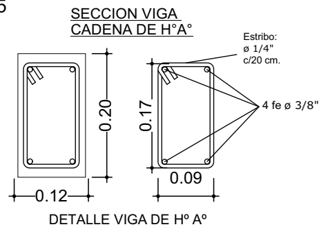
4 PLANO DE VIGA ENCADENADO
