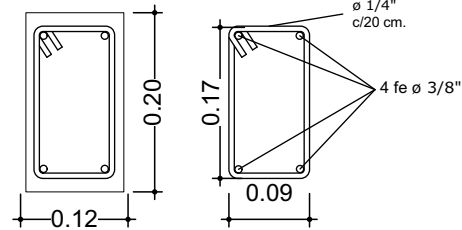
SECCION VIGA CADENA DE H°A°
