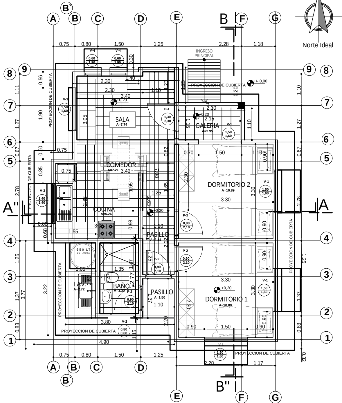
PLANTA ACOTADA ESC. 1:75
