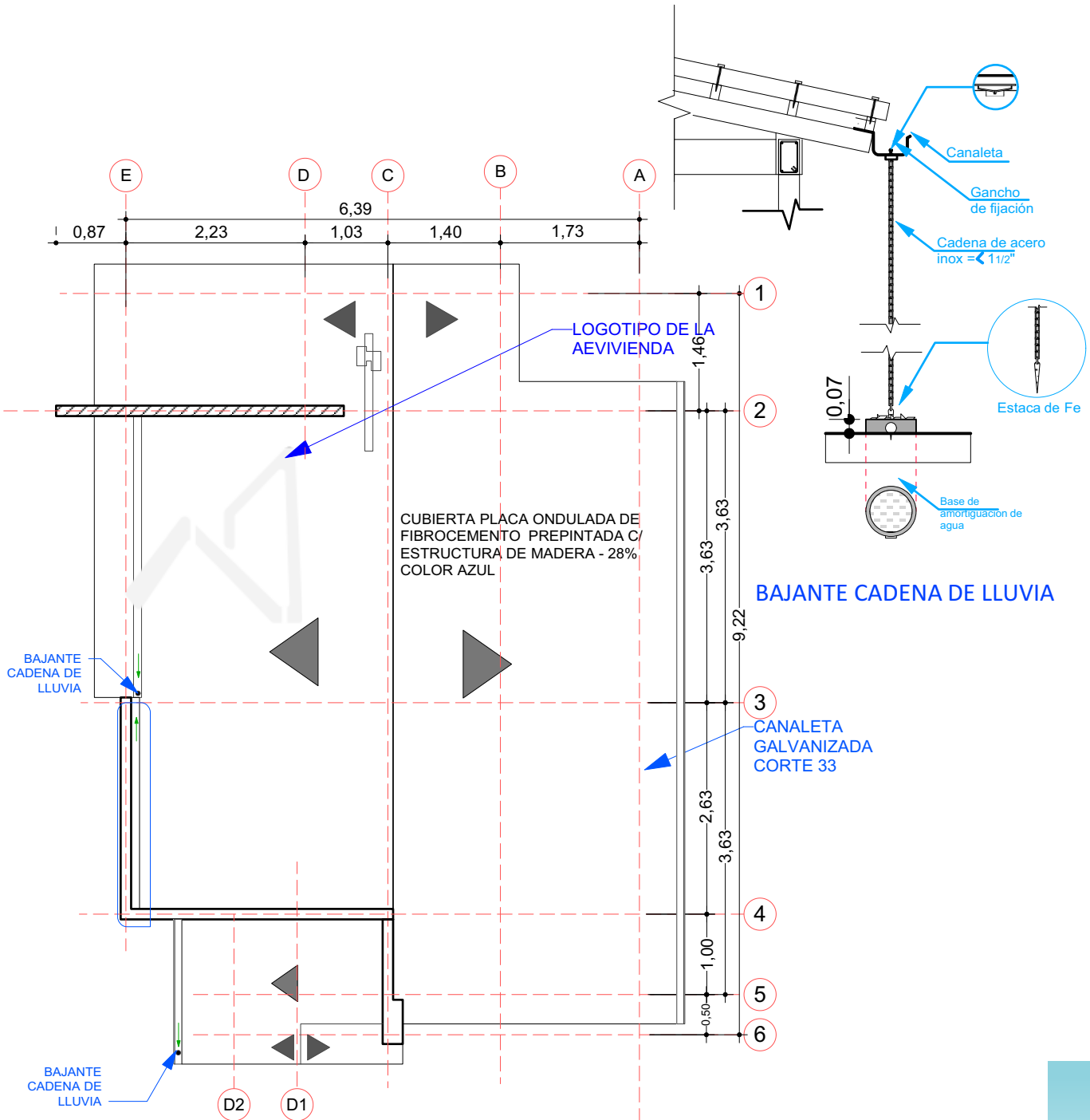
7 PLANO DE CUBIERTA
