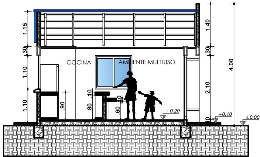
CORTE A-A' ESCALA: 1:75
