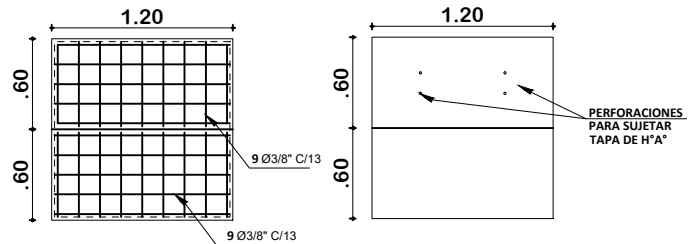
PLANTA
