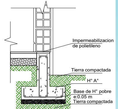
SECCION ESTRIBO
