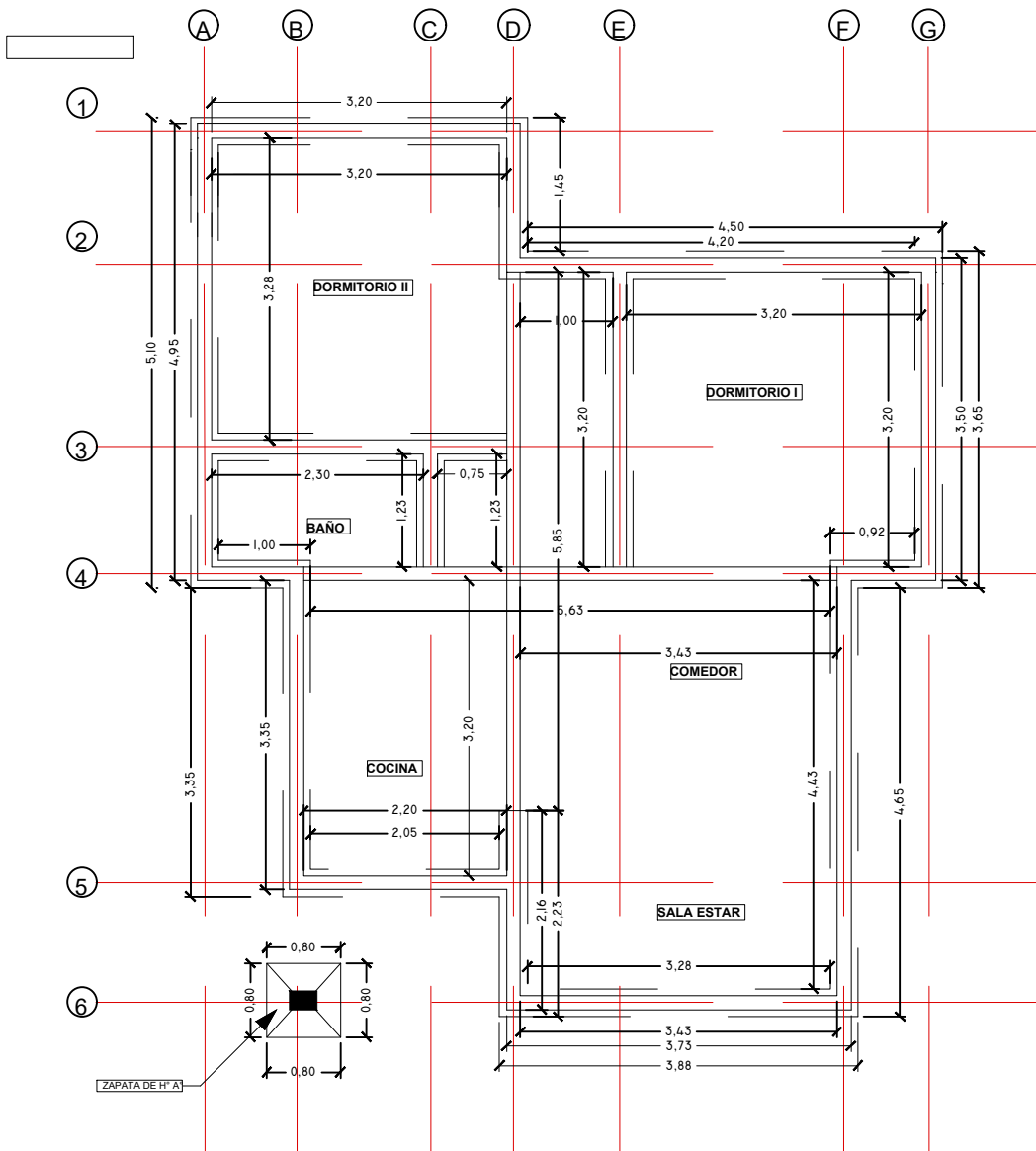
PLANO ESTRUCTURAL DE FUNDACION ESC.: 1:75
