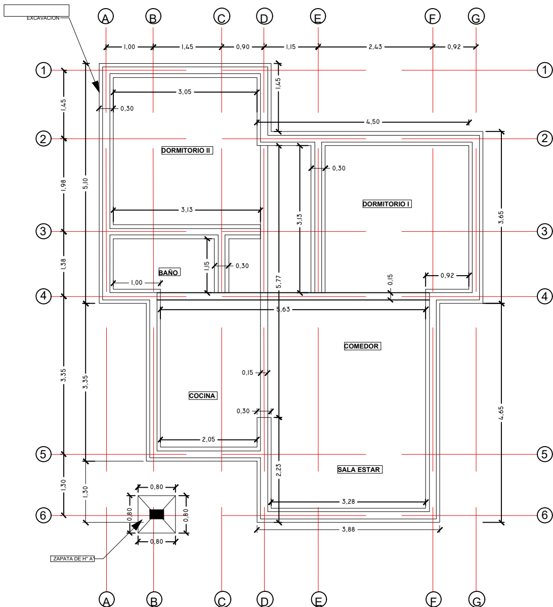
PLANO DE EXCAVACION ESC.: 1:75
