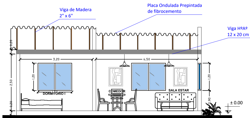
CORTE LOGITUDINAL B - B ESC.: 1:75
