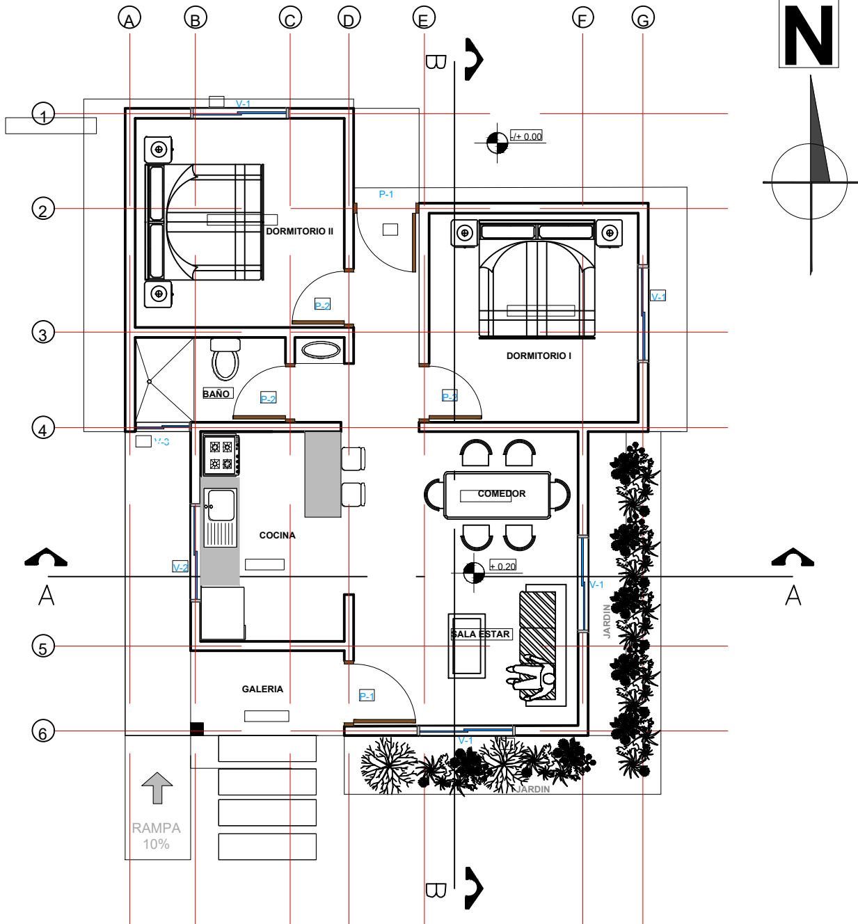
PLANTA AMOBLADA GENERAL ESC 1:75
