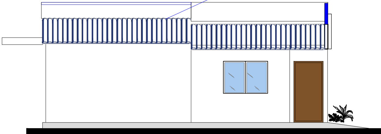
FACHADA LATERAL DERECHO ESC.: 1:75
