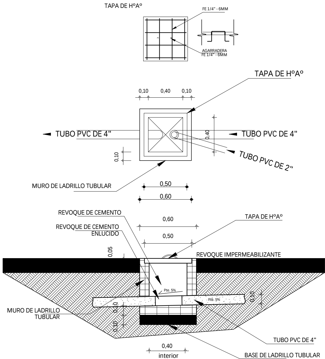
DETALLE CAMARA DE INSPECCION ESC. 1:35
