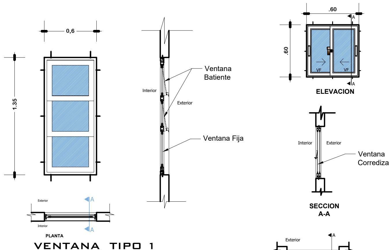
DETALLE VENTANA DE ALUMINIO 0.60x1.35
