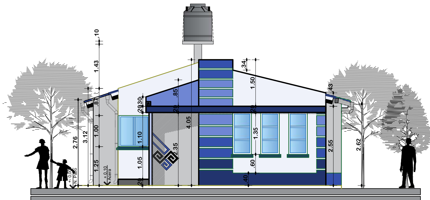
ELEVACION FRONTAL
