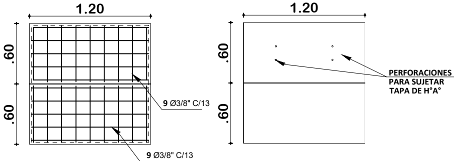
PLANTA
