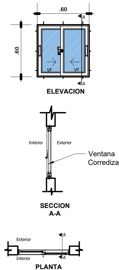
DETALLE VENTANA DE ALUMINIO 0.60x0.60
