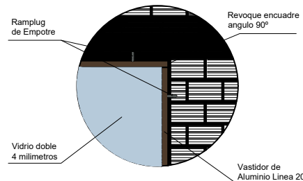
DETALLE VENTANA DE ALUMINIO LINEA 20 C/VIDRIO 4MM + ACCESORIOS
