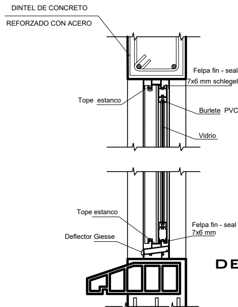
DETALLE VENTANA DE ALUMINIO 0.60x1.35
