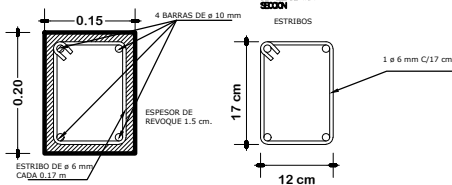
DETALLE DE VIGA 15x20
