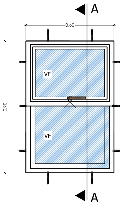
ELEVACION
