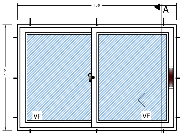
ELEVACION
