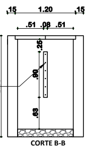
CORTE B-B
