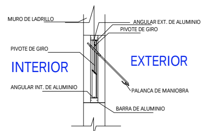
SECCION A - A'
