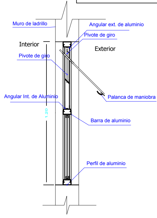
SECCION A-A
