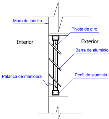
SECCION A-A
