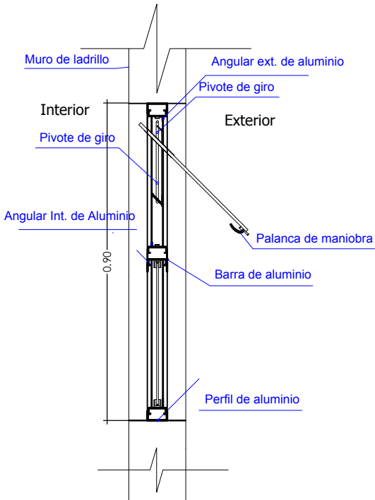
SECCION A-A
