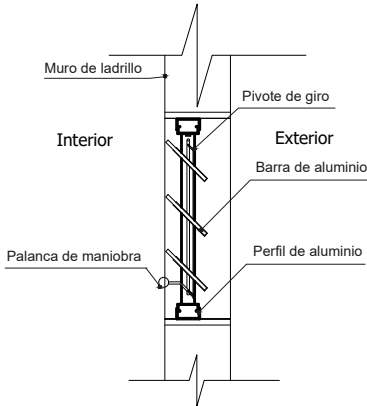
SECCION A-A
