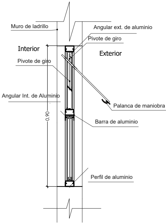
SECCION A-A
