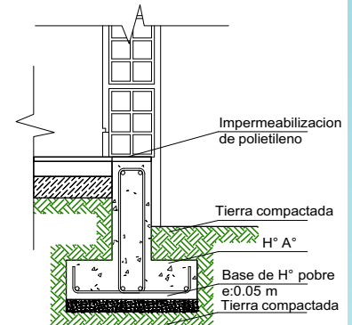
SECCIÓN ESTRIBO
