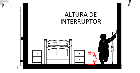
CORTE REFERENCIAL
