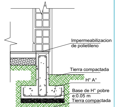
SECCIÓN ESTRIBO
