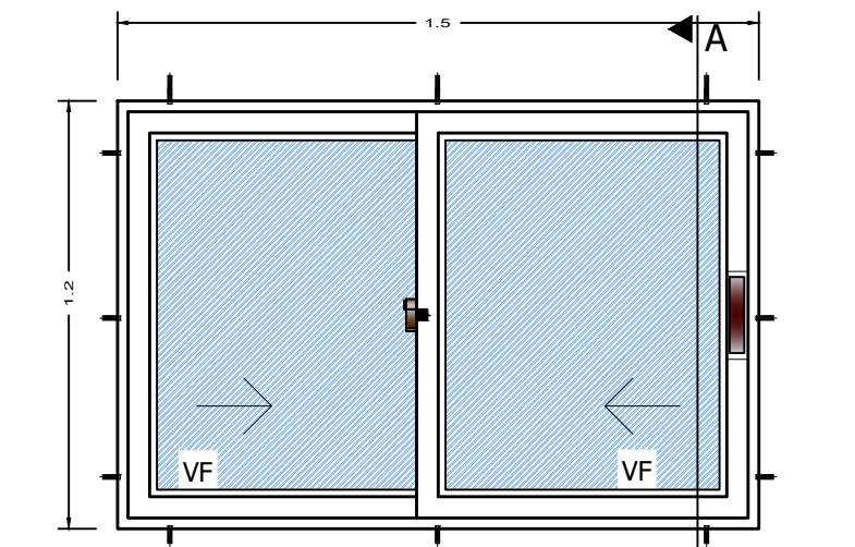
ELEVACION
