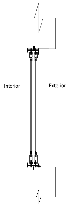
SECCION A-A
